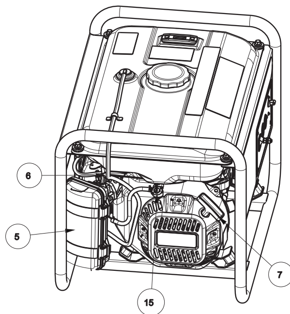
Figure 2 - Commandes générateur/moteur
