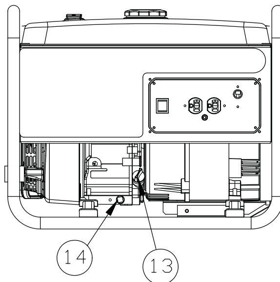
Figure 3 - Commandes générateur/moteur
